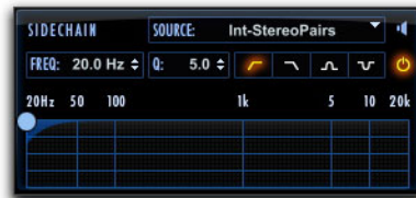
Side-Chain section
